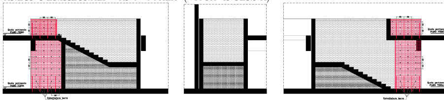
PARETI PERIMETRALI VANO SCALA (VISTA INTERNA)
