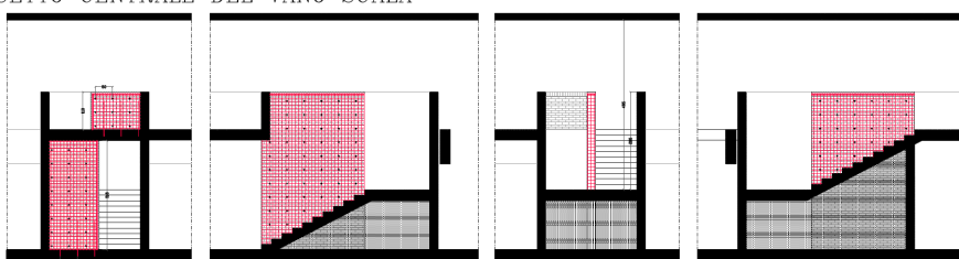
SETTO CENTRALE DEL VANO SCALA
